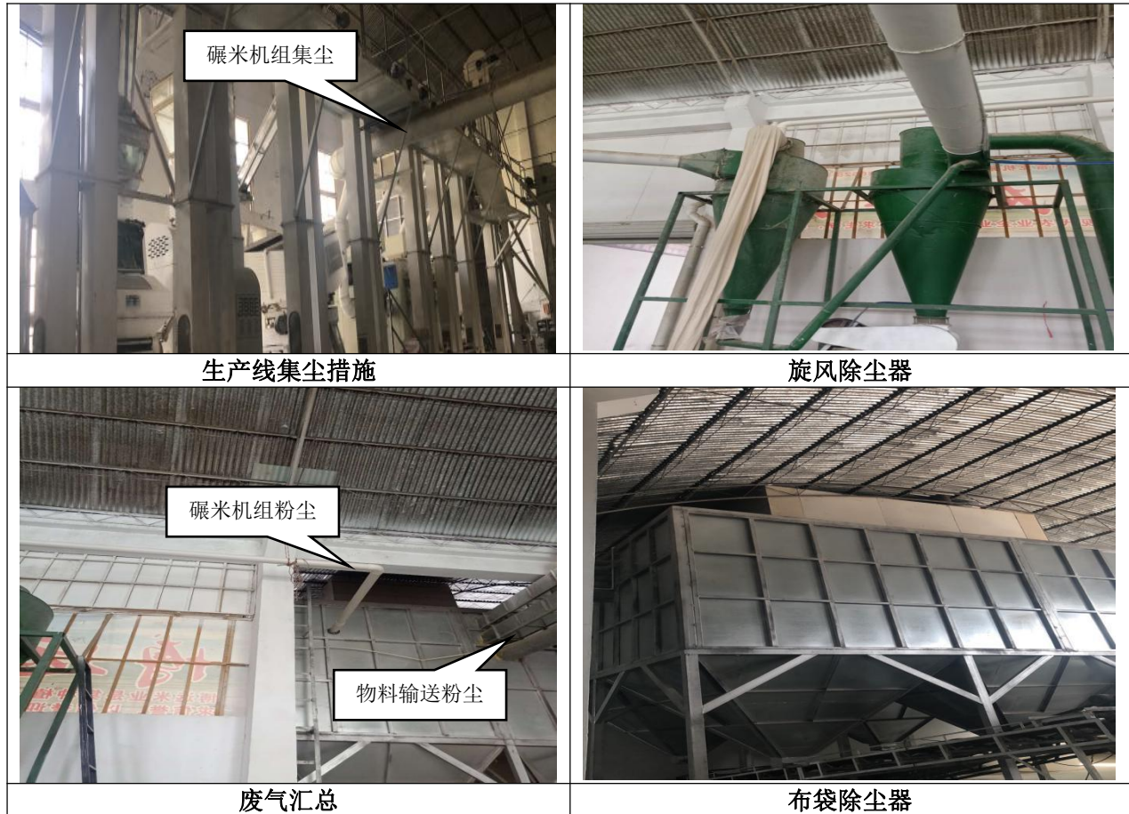
图 4-2 项目废气治理流程图
