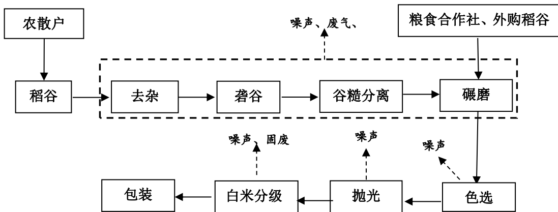
图 3-4 项目工艺流程图
