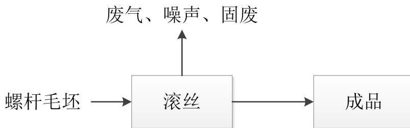
图 3-4 滚丝螺杆工艺流程
